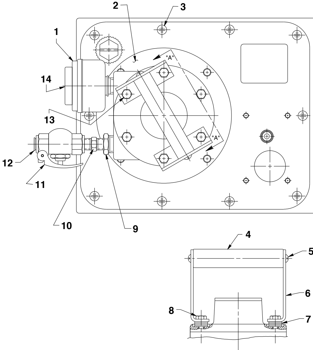
VIEW A-A
